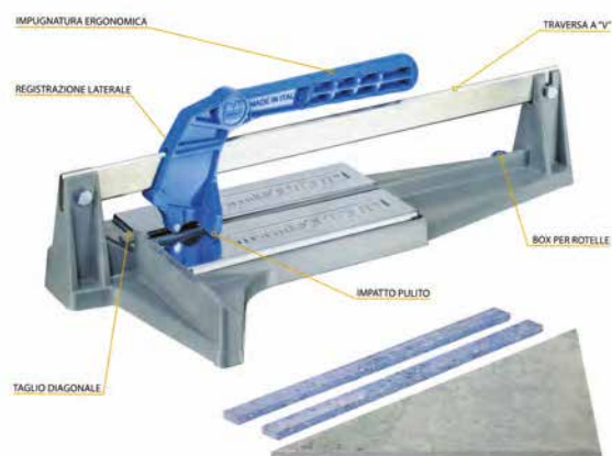
Tagliapiastrelle "Minimontolit"
