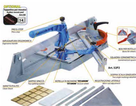
Tagliapiastrelle "Masterpiuma"
