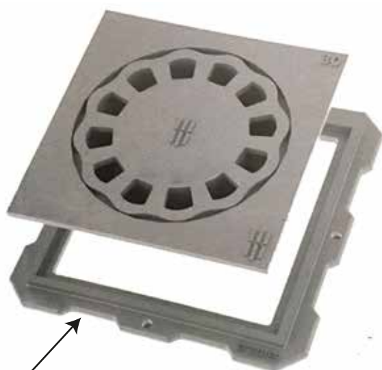
Telaio optional per 30x30 e 40x40
